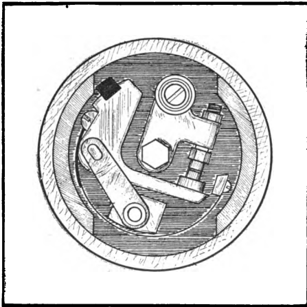
MAGNETO BREAKER (Bosch).
